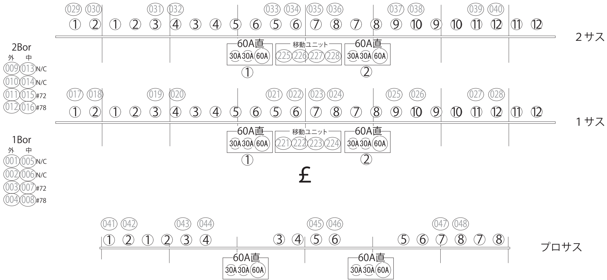
清水マリナート 小ホール SUS回路図
